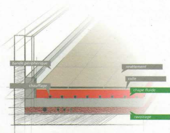
Ravoirage sous chape flottante et système de chauffage par le sol.
